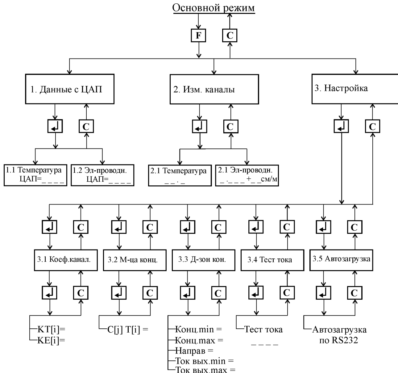
Рисунок А.1 - Структура пунктов настройки и управления прибором
