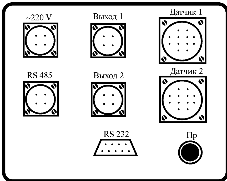
Рисунок А.2 – Вид лицевой панели электронного блока
